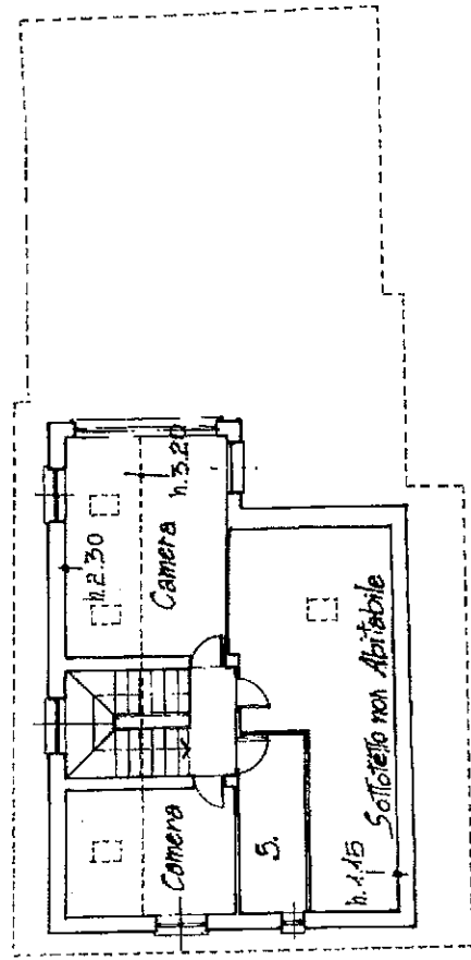
Piano Sottotetto
